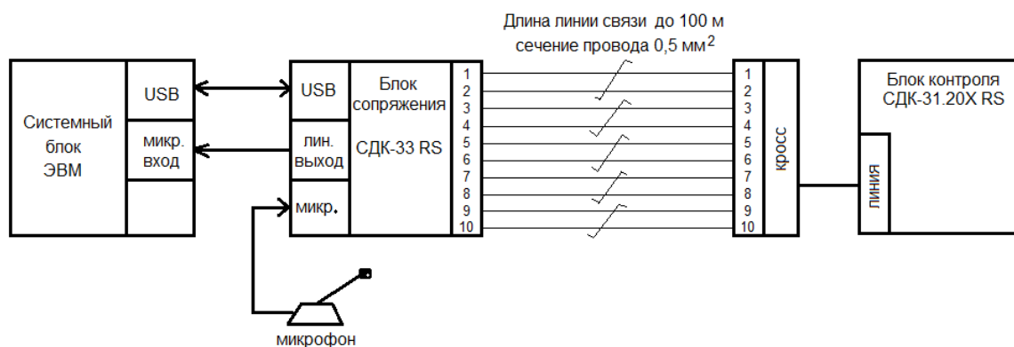
Рисунок 1. Схема подключения блока сопряжения СДК-33RS
