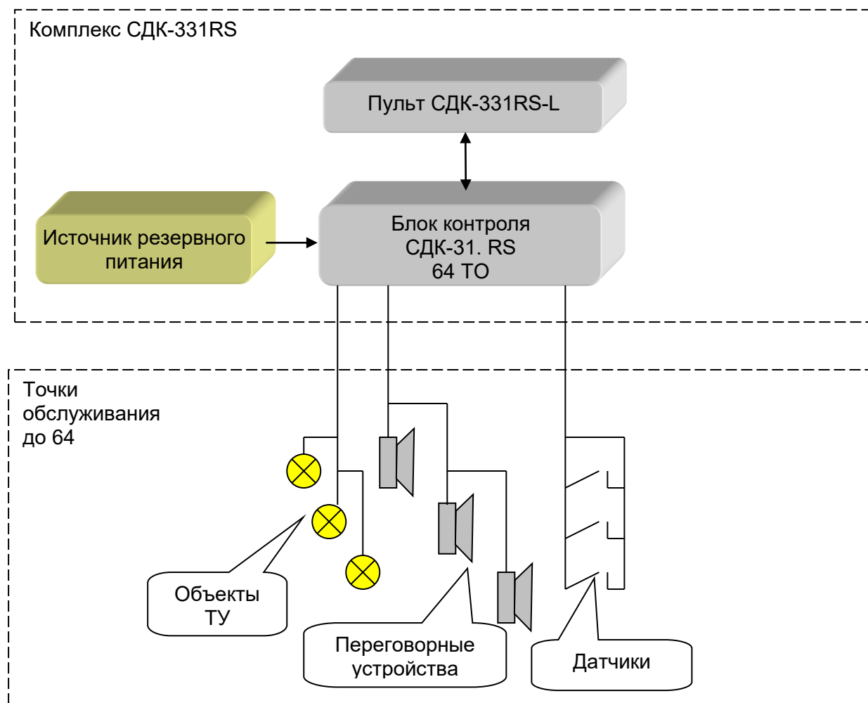
Рисунок 1. Система диспетчеризации на базе комплекса СДК-331RS
