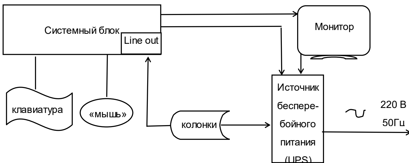
Рис.2. Схема соединений компьютера пульта диспетчера
