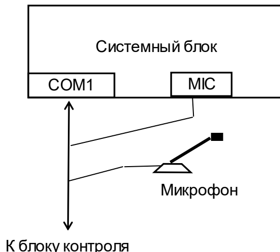
Рис.5. Схема подключения пульта диспетчера СДК-330RS
