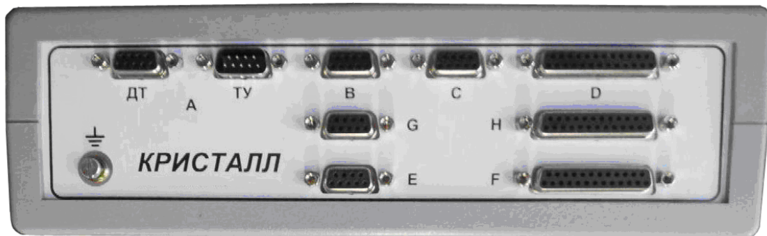
Рис. 1. Расположение разъемов на блоках СДК 31.x05, СДК 31.x08, СДК 31.x09, СДК 31.x18, СДК 31.x19.
