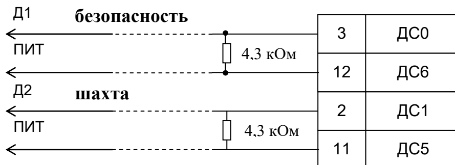
Рис. 17. Подключение к доработанной станции управления УЛ-30Пп (установлены реле дополнительных сигналов диспетчеризации).
