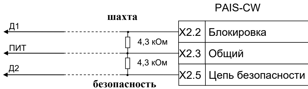
Рис. 13. Подключение для снятия сигнала безопасности и открытия дверей шахты к станции управления фирмы «ОТИС»
