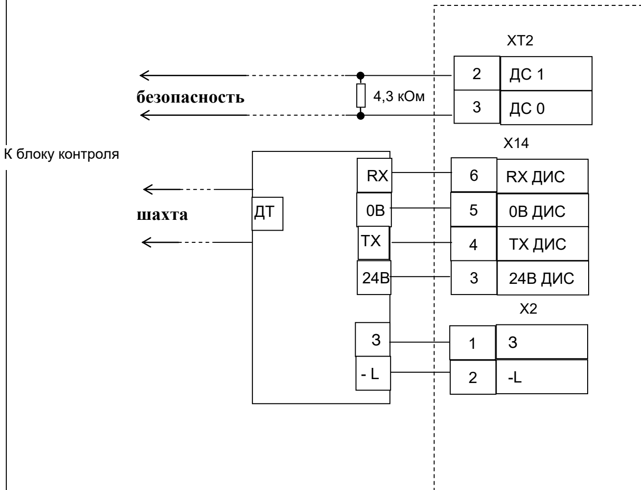
Рис. 16. Подключение для снятия сигналов безопасности и проникновения в шахту к станции управления УЛ
