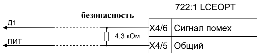
Рис 14. Подключение для снятия сигнала безопасности станции управления лифтом фирмы «КОНЕ».
