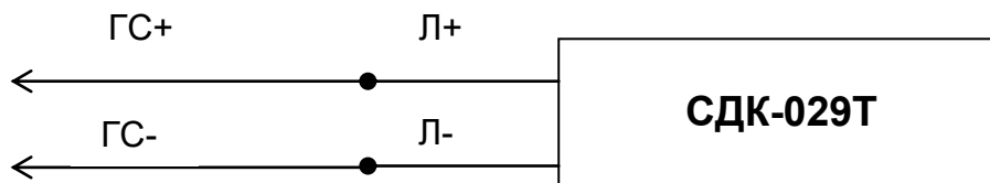
Рис. 6а. Подключение СДК-029Т
