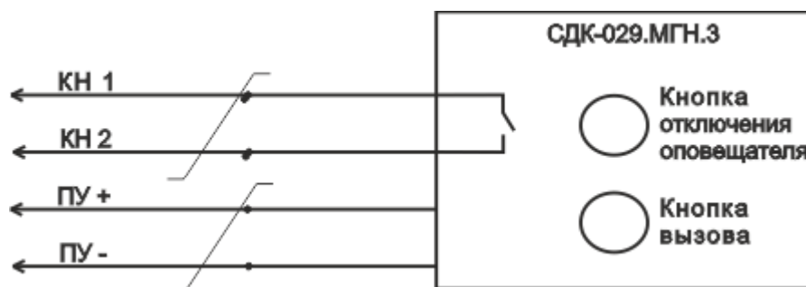
Рис. 3. Подключение СДК-029.МГН.3
