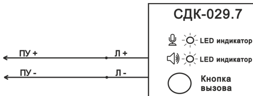
Рис. 3. Подключение СДК-029.7
