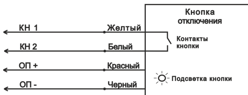
Рис. 5. Подключение кнопки отключения оповещателя
