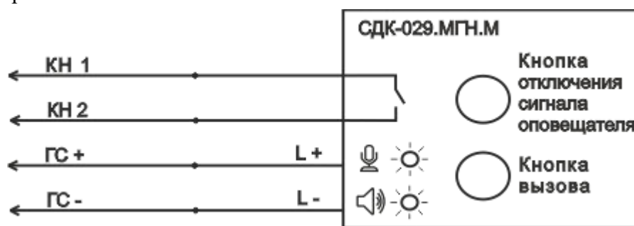
Рис. 1. Подключение СДК-029.МГН.М
