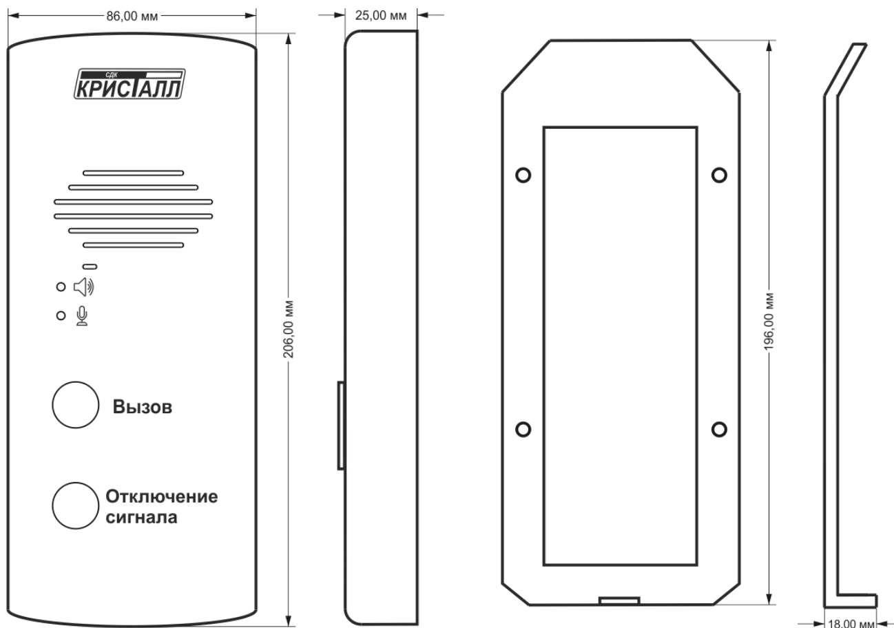
Рис. 2. Корпус СДК-029.МГН.М с монтажной пластиной.
