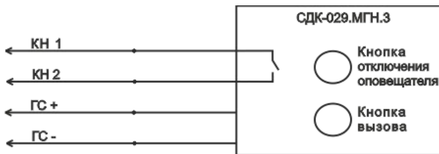
Рис. 1. Подключение СДК-029.МГН.3
