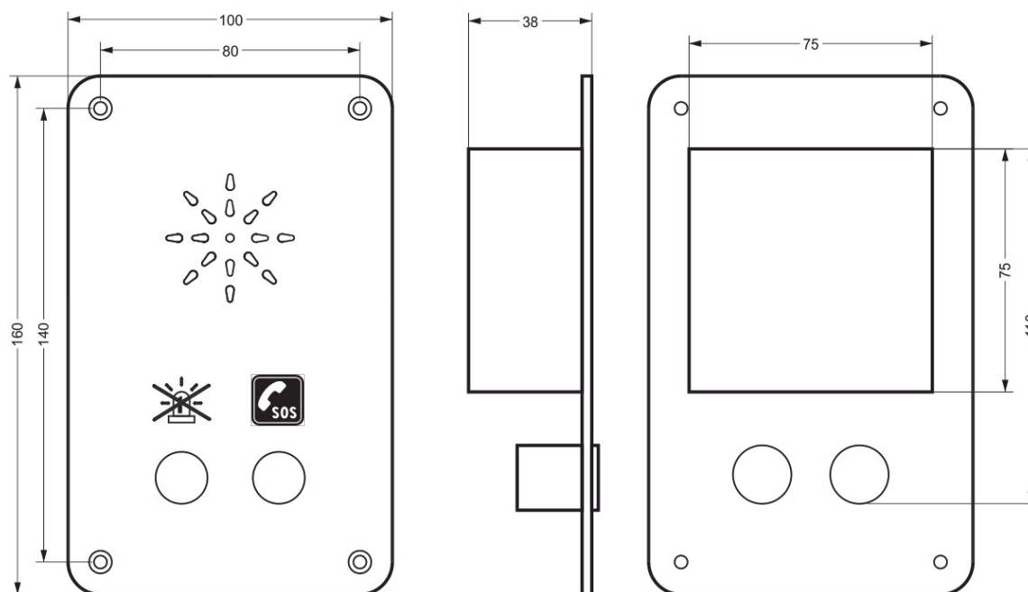
Рис. 2. Габаритные размеры СДК-029.МГН.3
