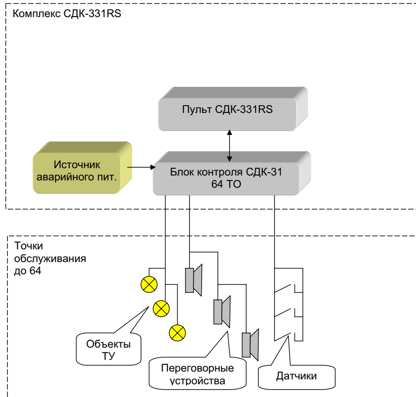
Рисунок 1. Система диспетчеризации на базе комплекса СДК-331RS
